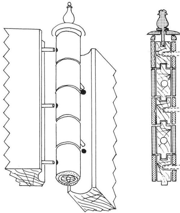
Exemple de montage des éléments de charnière.
